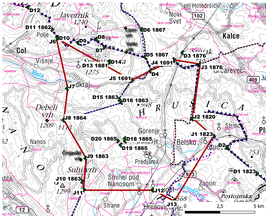
Slika 4: Zeleni rombi so lokacije, obravnavane v članku: J iz preglednice 1, D iz preglednice 2, lokacije brez številke so v besedilu zgolj omenjene (podlaga: DPK 1 : 250.000, GURS).
