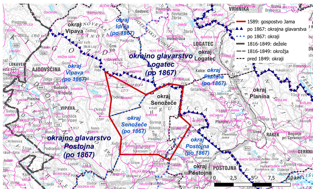
Slika 2: Nekdanje meje gospostva Jama iz leta 1589 (rdeča), dežel, okrožij in okrajev med letoma 1816 in 1849 (sivo črtkano in pokončni sivi napisi), okrajnih glavarstev in okrajev po letu 1867 (modri trikotniki in ležeči modri napisi) in današnje meje katastrskih občin (rožnate). Prikazane meje so le informativne narave (podlaga: DPK 1 : 250.000, GURS).
