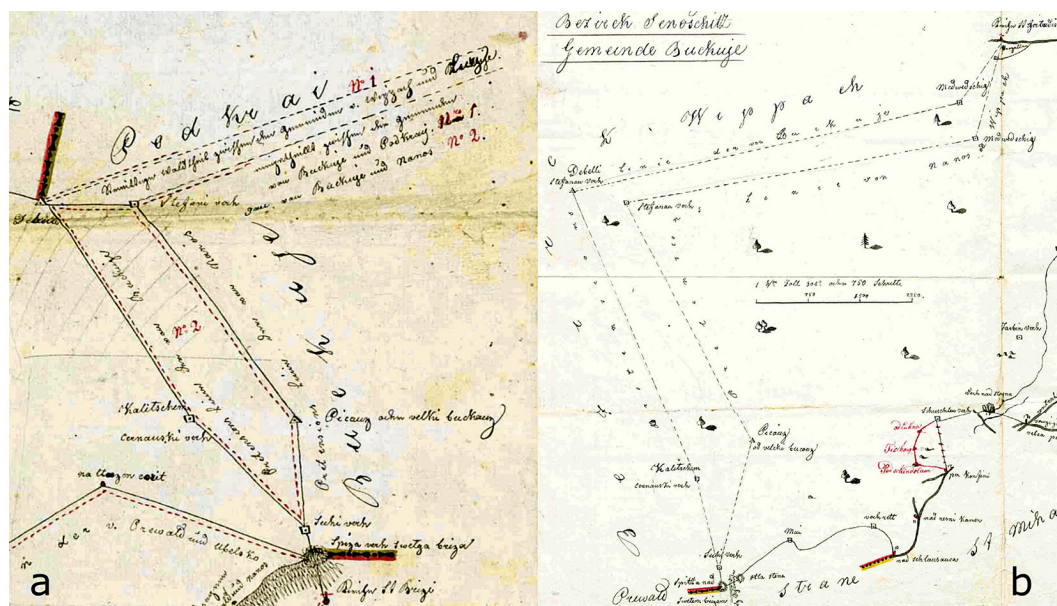
Slika 3: Deli mej katastrskih občin pod Podkrajem, ki so med franciscejsko izmero leta 1824 imele še dve varianti poteka. Izseka iz skic franciscejske zemljiškokatastrske izmere: a) katastrska občina Nanos (vir: SI AS 176/A/A20/s/PG, 1824) in b) katastrska občina Hrušica (vir: SI AS 176/A/A102/s/PG, 1823).
