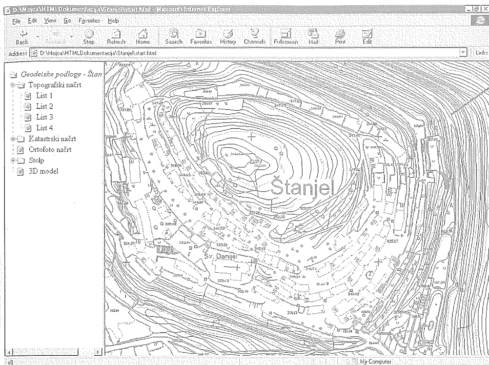
Slika 3: Topografski načrt Štanjela v merilu 1 : 1000
